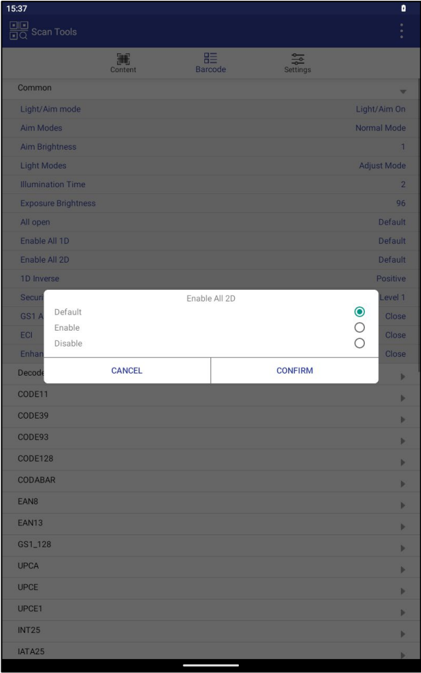
Рисунок 137. Barcode. Enable All 2D
