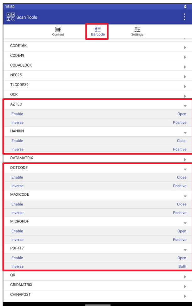
Рисунок 165. AZTEC, HANXIN, DOTCODE, MAXICODE, MICROPDF, PDF417
