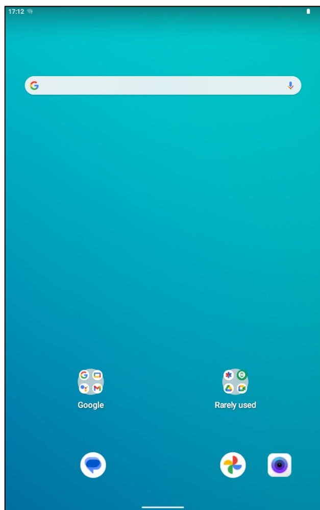
Рисунок 9. Главный экран
