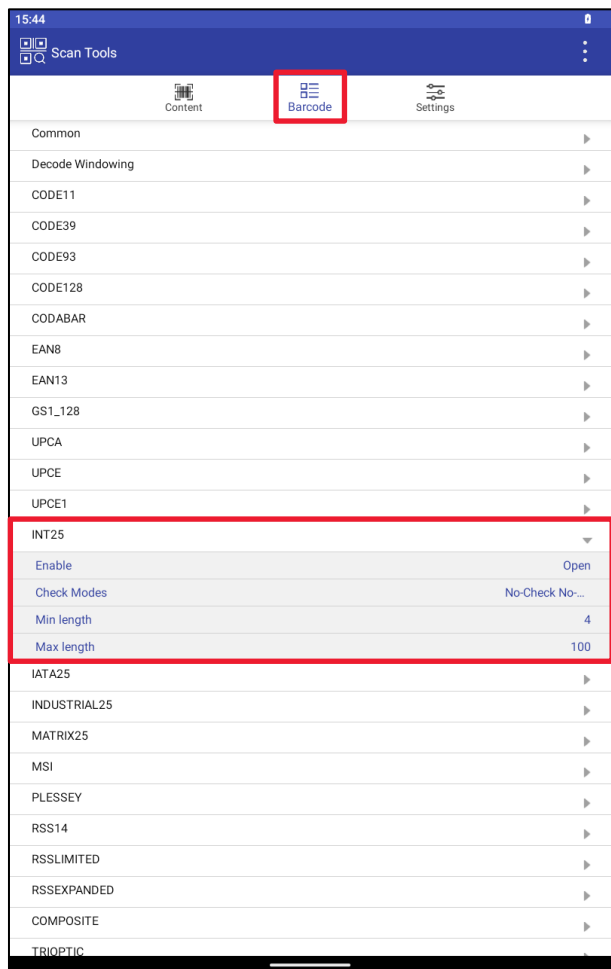
Рисунок 154. INT25
