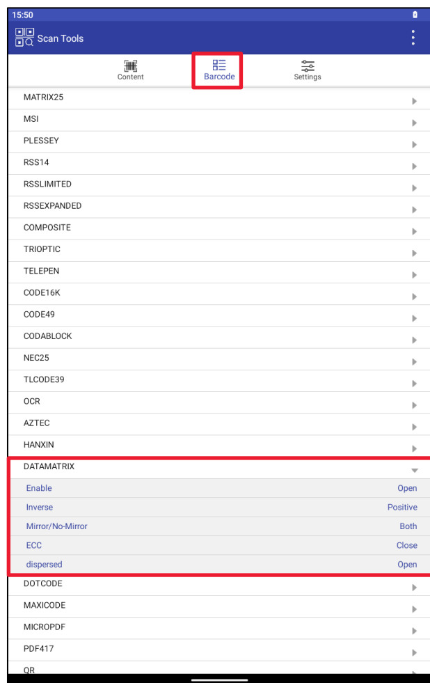
Рисунок 166. DATAMATRIX
