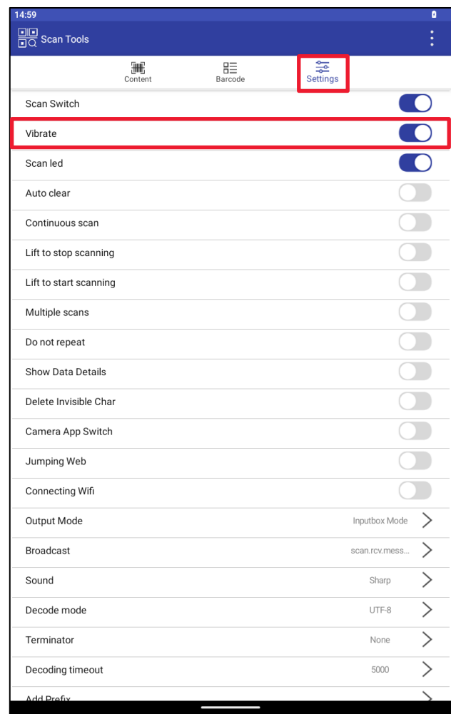
Рисунок 101. Settings. Vibrate
