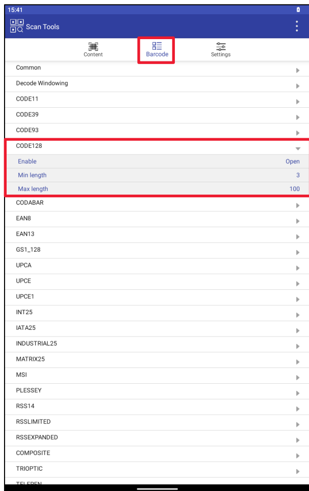
Рисунок 146. CODE128
