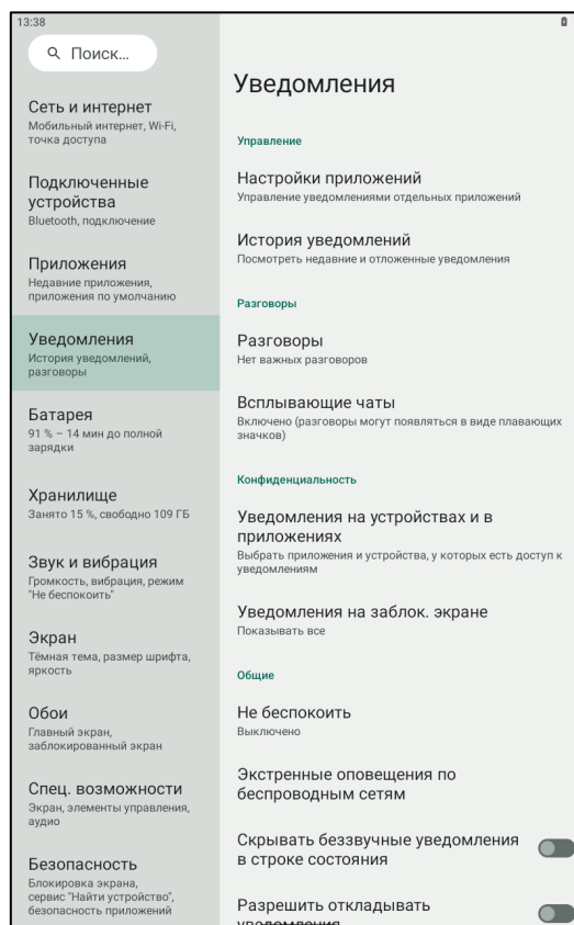
Рисунок 27. Уведомления
