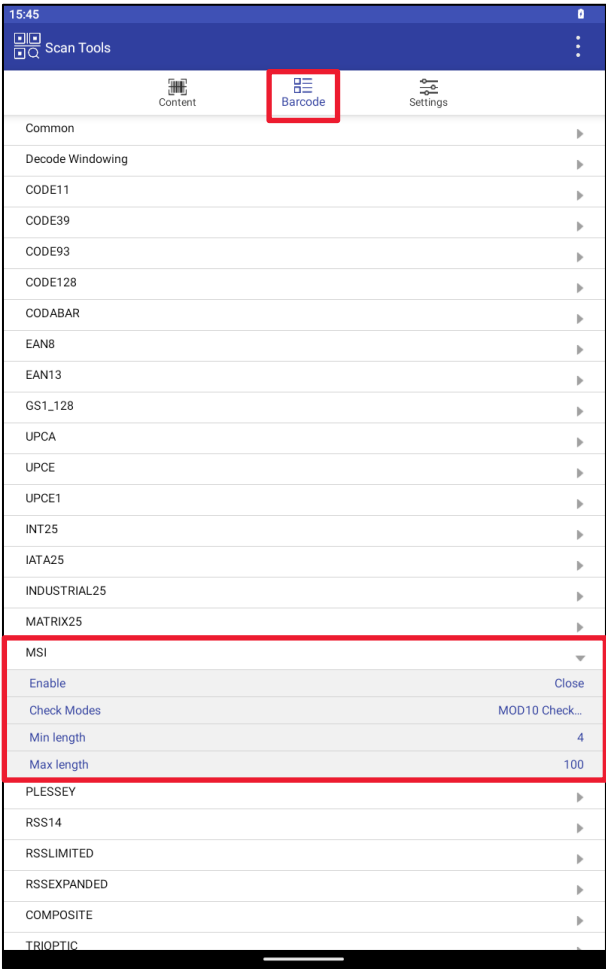
Рисунок 158. MSI
