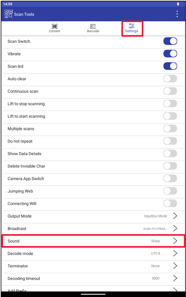
Рисунок 120. Settings. Sound
