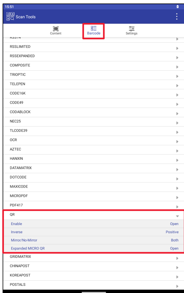
Рисунок 167. QR
