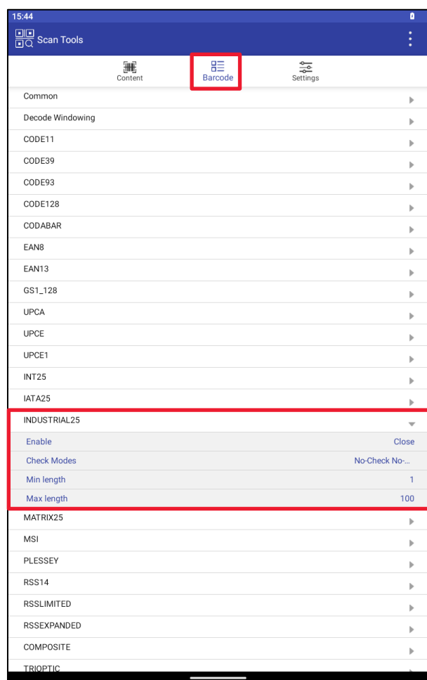
Рисунок 156. INDUSTRIAL25
