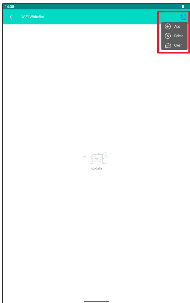
Рисунок 89. WIFI Whitelist
