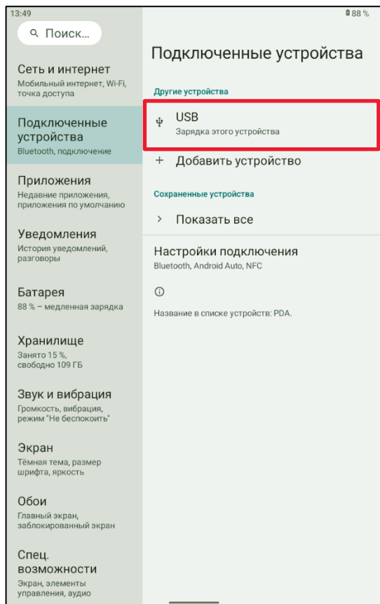
Рисунок 173. Подключенные устройства
