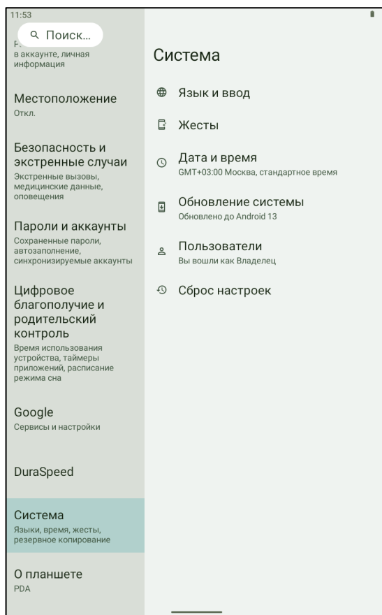
Рисунок 48. Система
