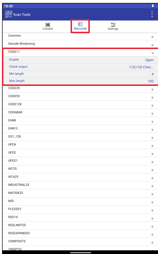
Рисунок 143. CODE11
