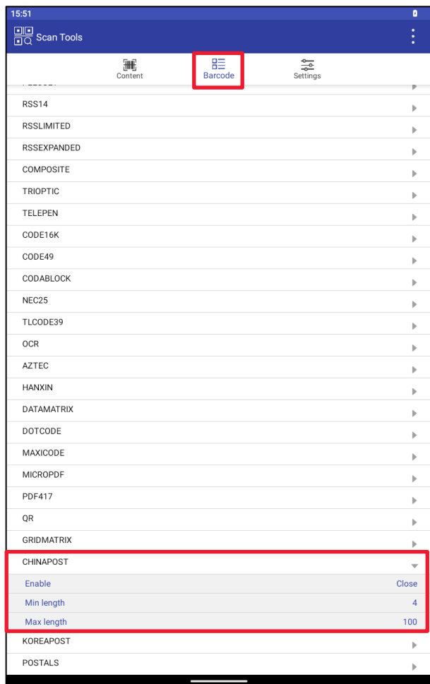
Рисунок 169. CHINAPOST
