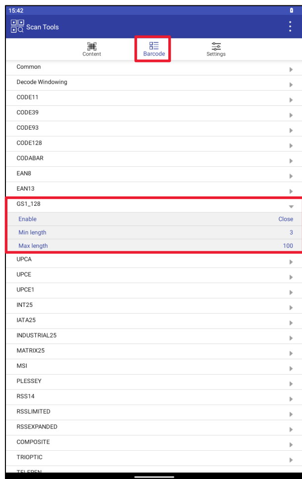
Рисунок 150. GS1_128
