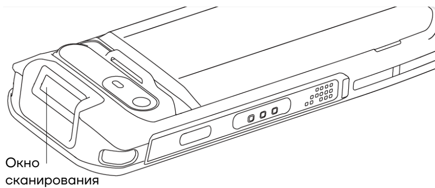
Рисунок 172. Окно сканирования
