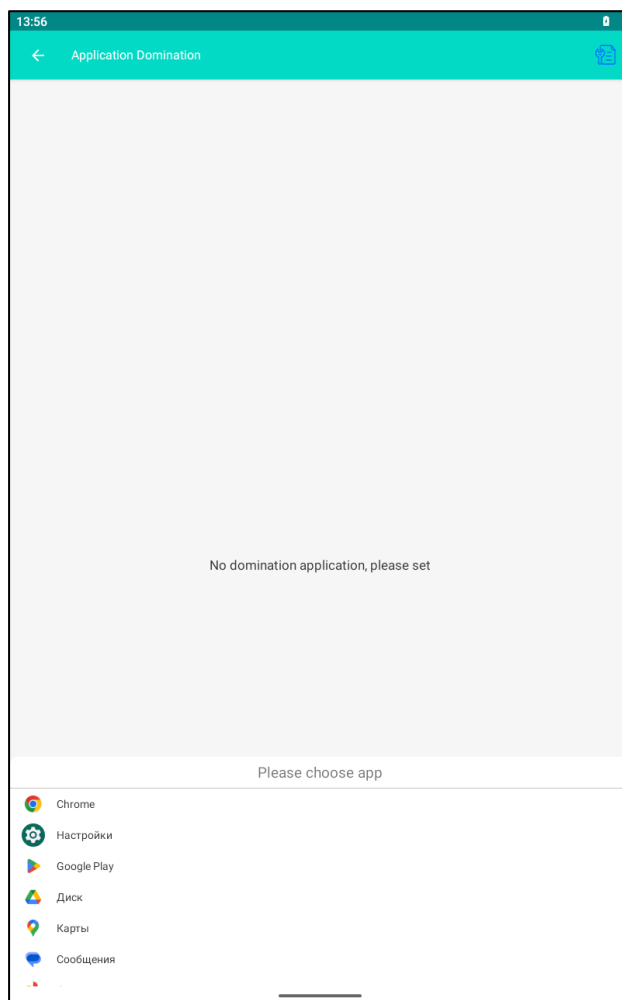
Рисунок 68. Application Domination
