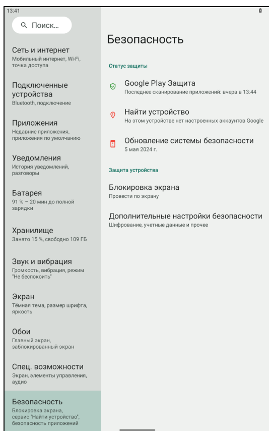
Рисунок 38. Безопасность
