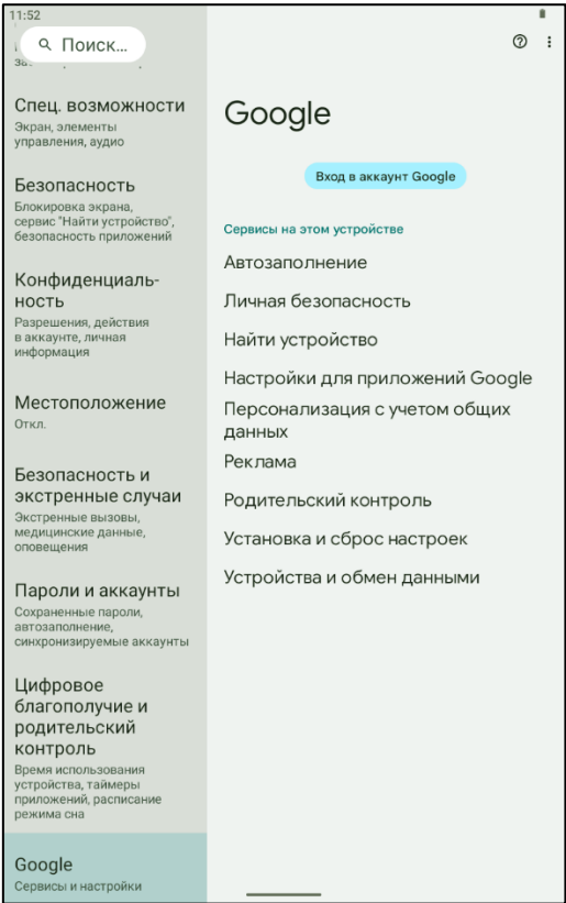
Рисунок 46. Google
