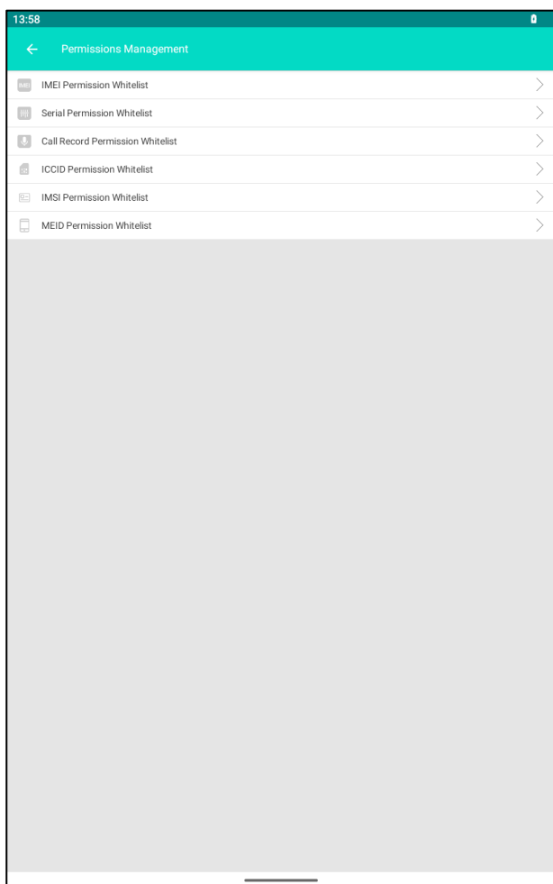
Рисунок 69. Permission Management
