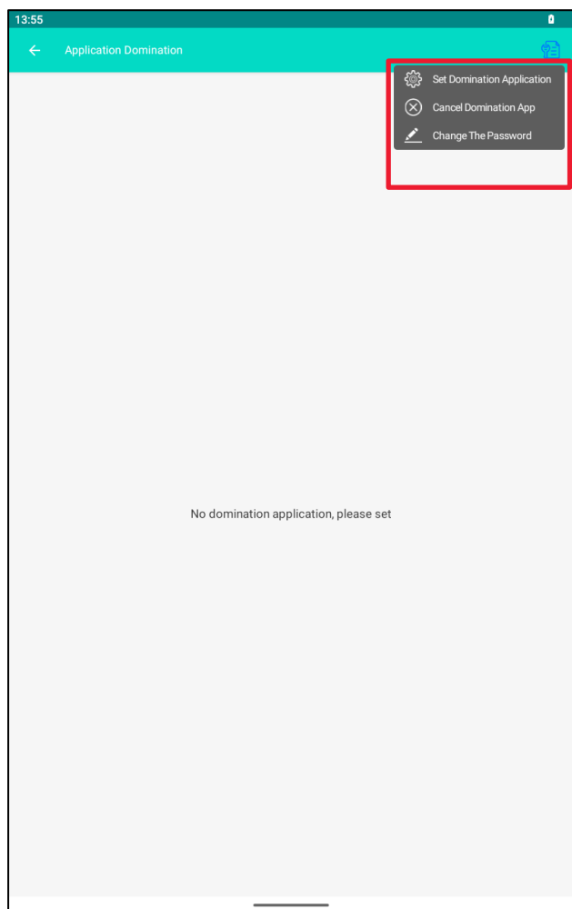
Рисунок 67. Application Domination
