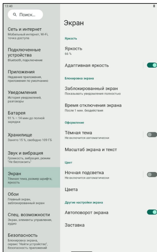
Рисунок 34. Экран
