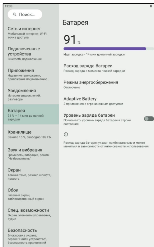
Рисунок 30. Батарея
