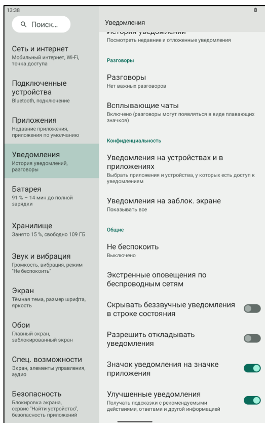
Рисунок 28. Уведомления. Продолжение
