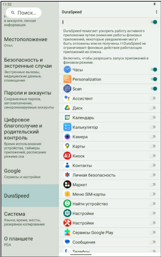
Рисунок 47. DuraSpeed
