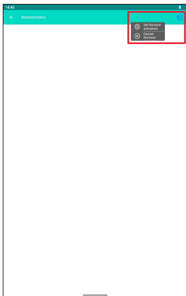
Рисунок 94. BootAnimation
