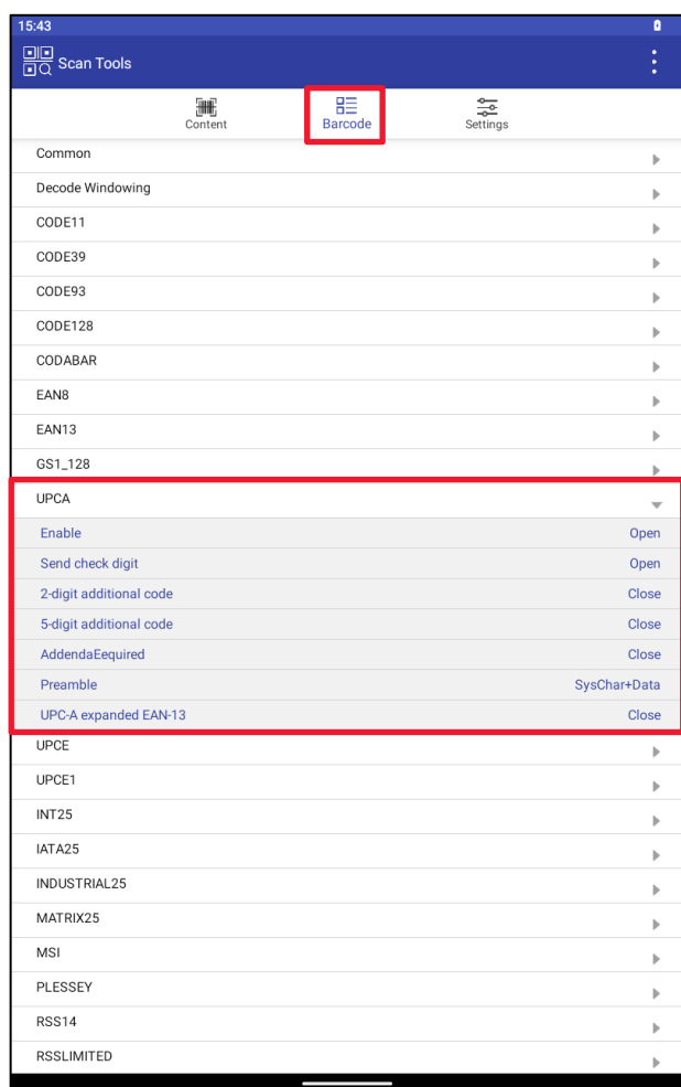
Рисунок 151. UPCA
