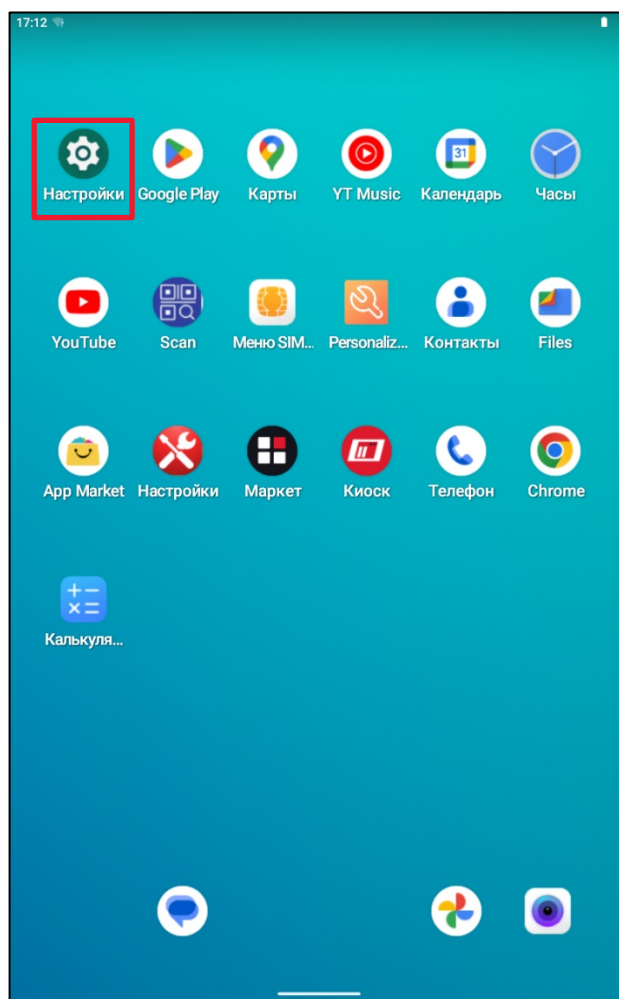
Рисунок 10. Список приложений
