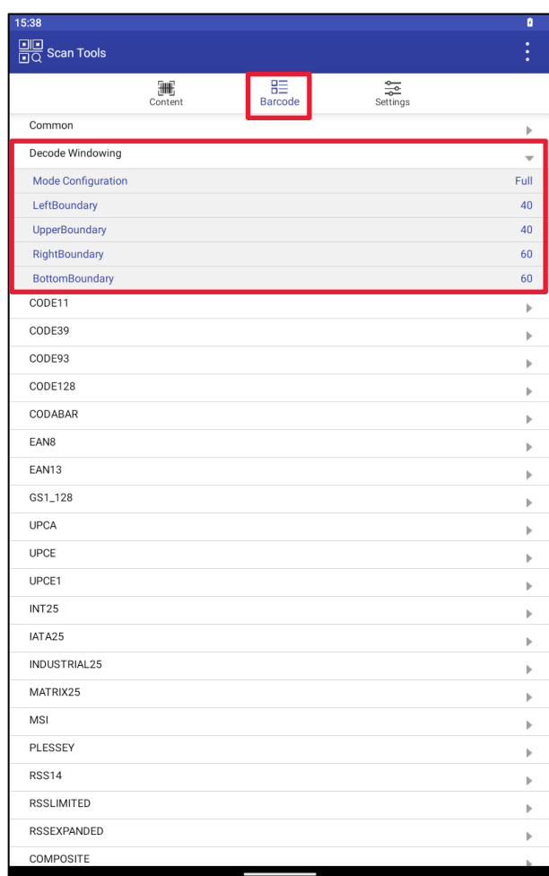
Рисунок 142. Barcode. Decoding Window
