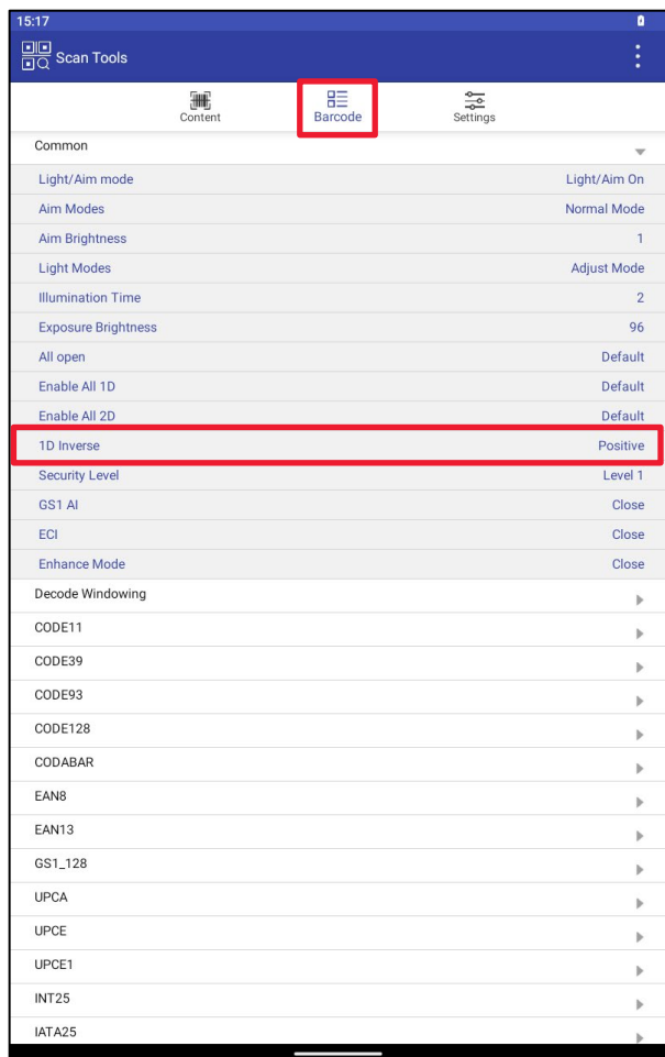
Рисунок 138. Barcode. 1D Inverse
