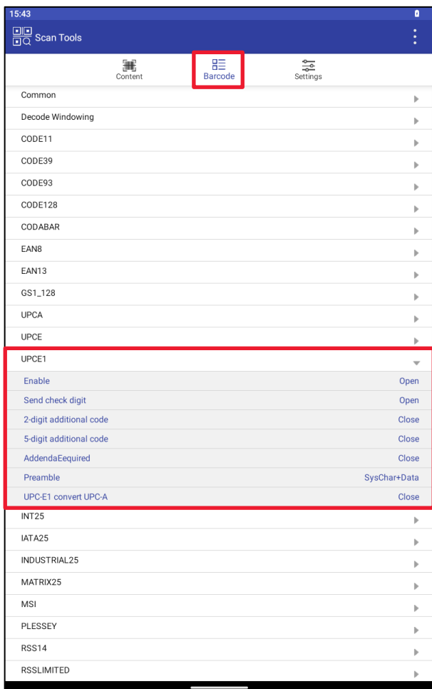
Рисунок 153. UPCE-1
