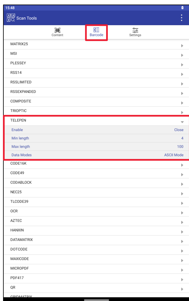
Рисунок 162. TELEPEN
