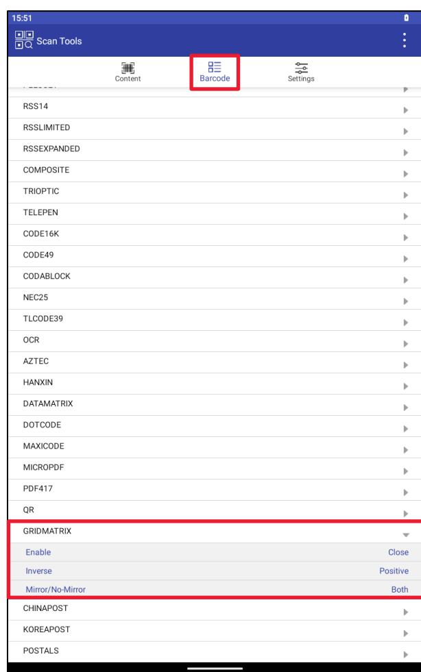
Рисунок 168. GRIDMATRIX
