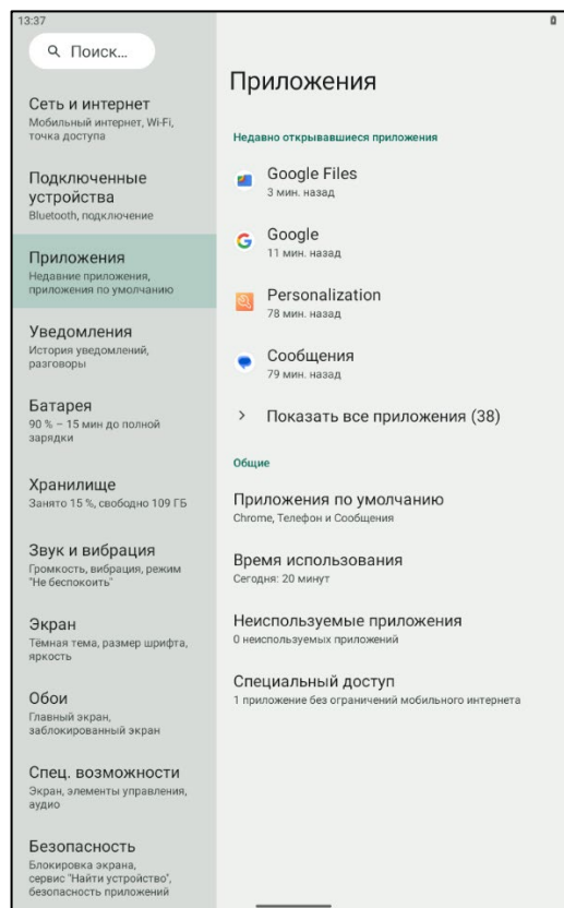
Рисунок 24. Приложения
