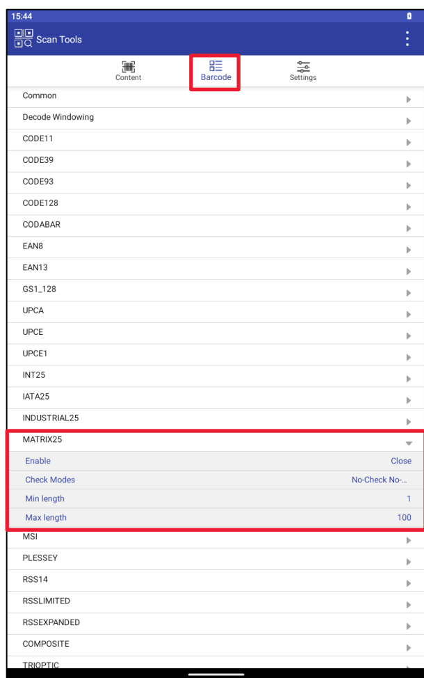
Рисунок 157. MATRIX25
