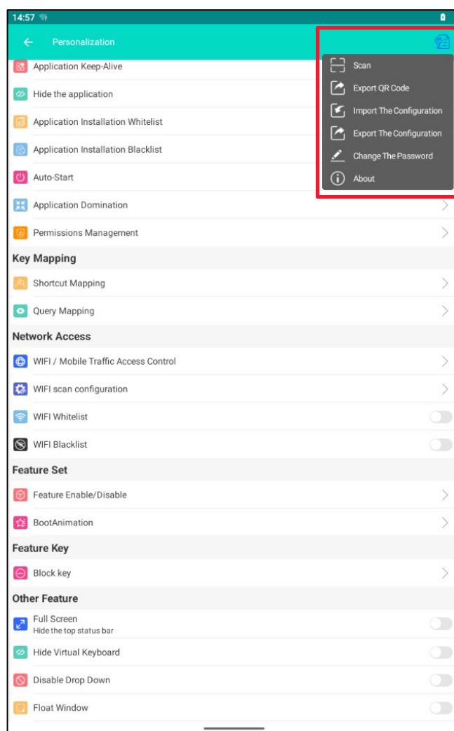
Рисунок 98. Personalization
