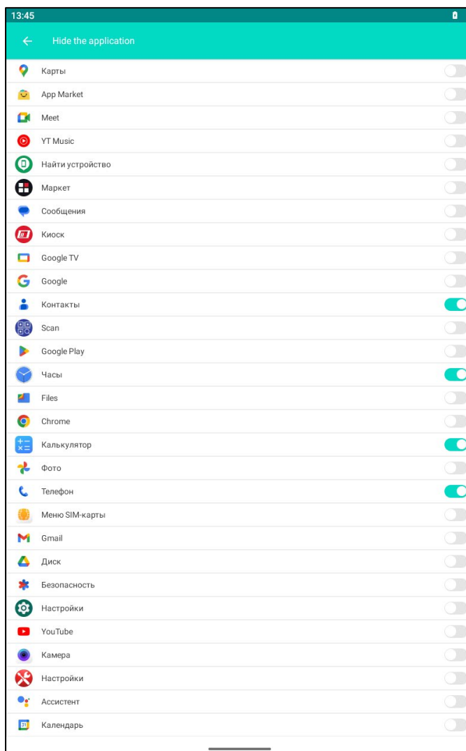
Рисунок 58. Hide application
