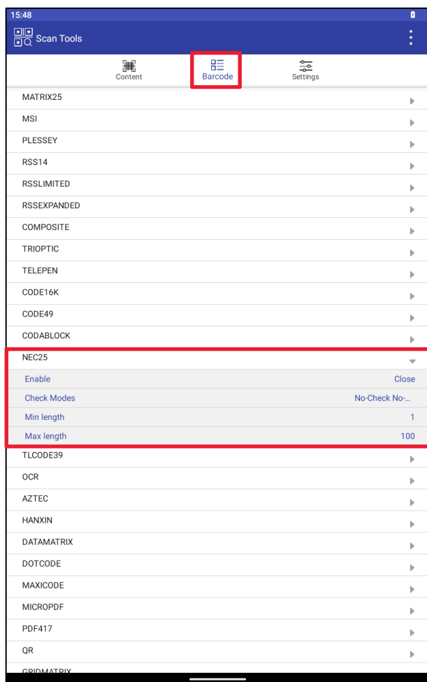
Рисунок 163. NEC25
