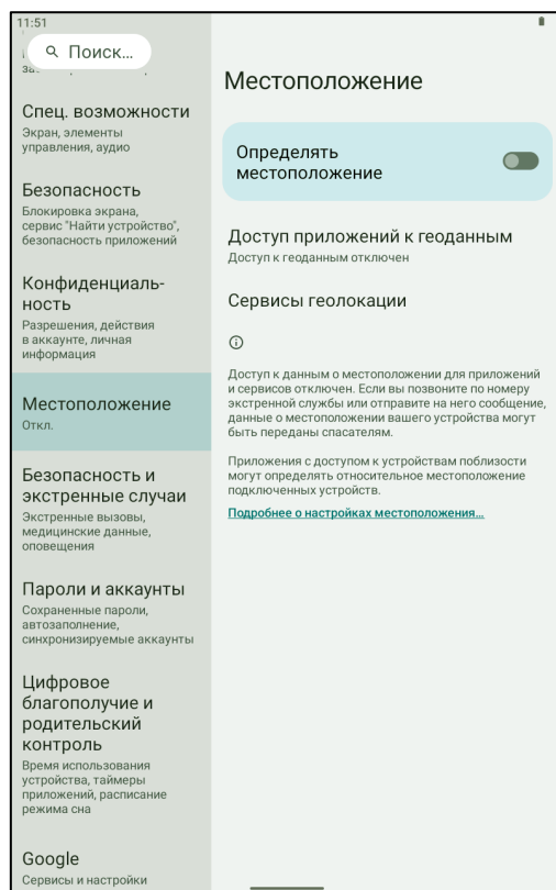
Рисунок 42. Местоположение
