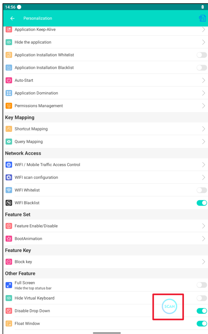
Рисунок 97. Другие функции
