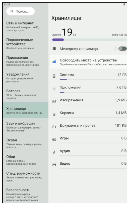
Рисунок 31. Хранилище
