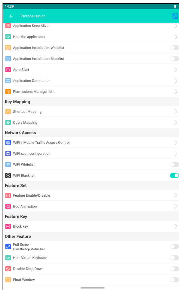
Рисунок 92. WIFI Blacklist
