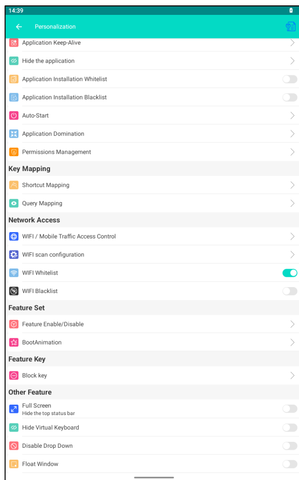
Рисунок 90. WIFI Whitelist
