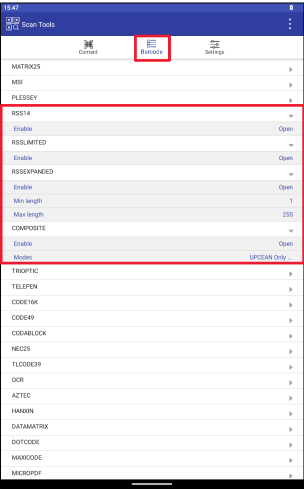
Рисунок 160. COMPOSITE
