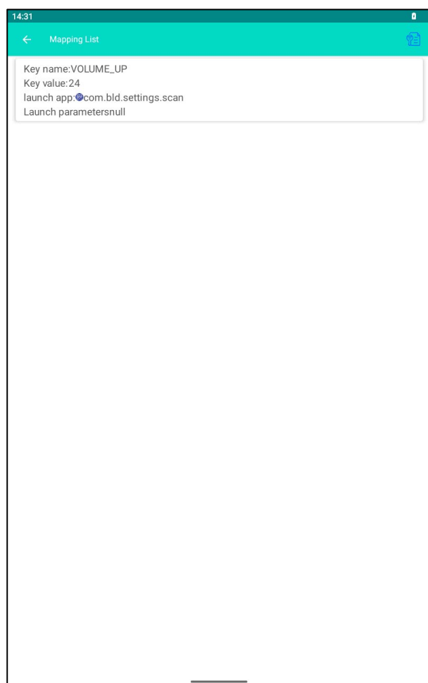
Рисунок 84. Query mapping
