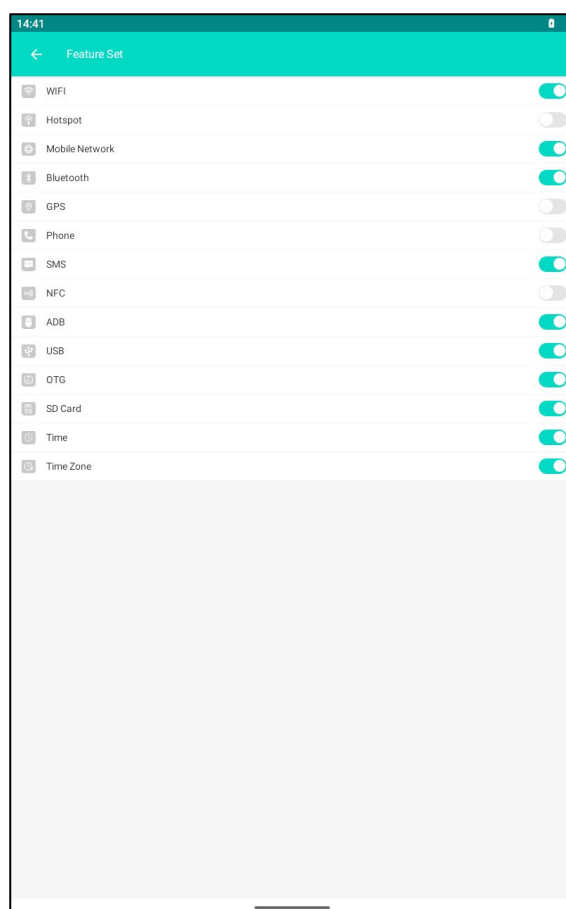
Рисунок 93. Feature Enable/Disable
