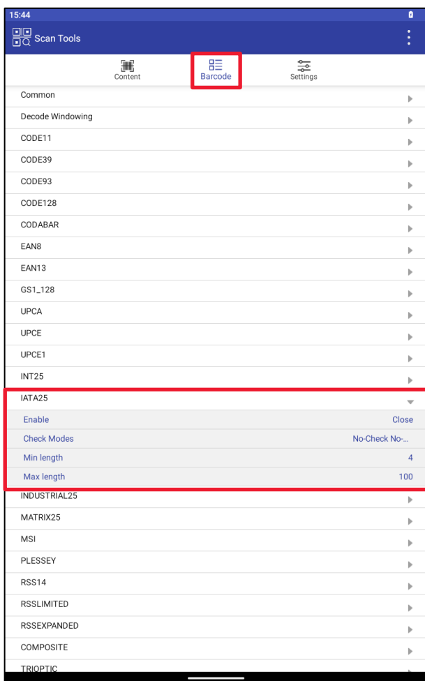
Рисунок 155. IATA
