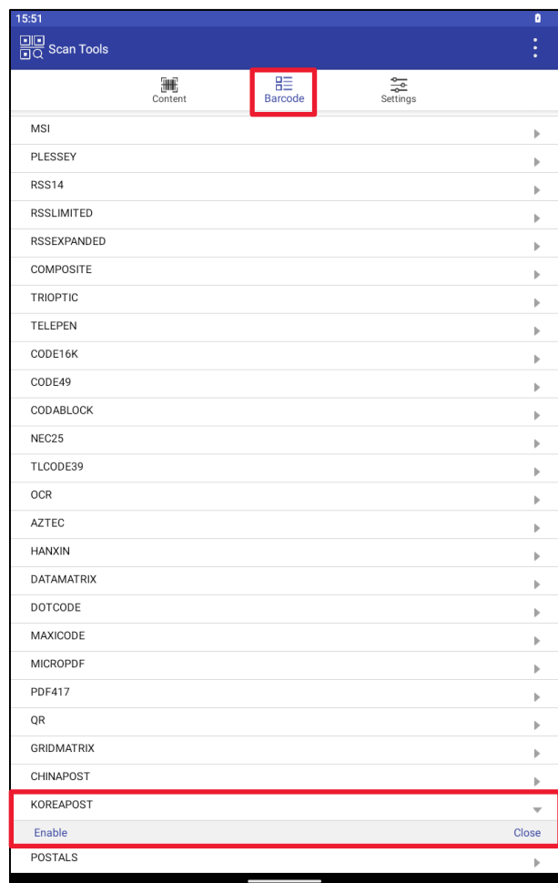
Рисунок 170. KOREAPOST
