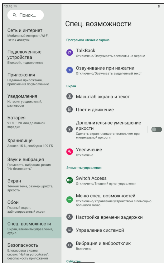
Рисунок 36. Спец. возможности
