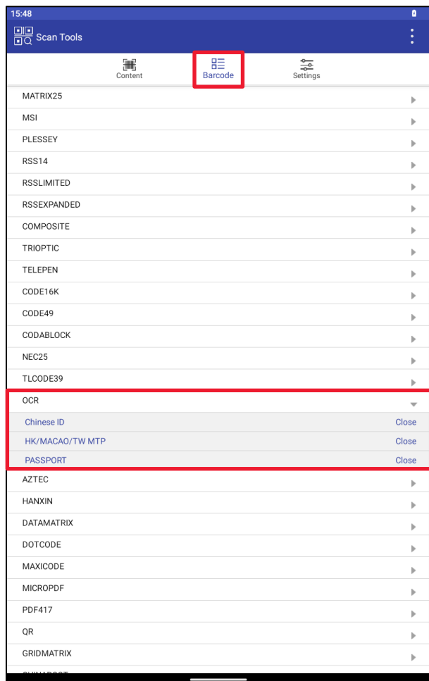
Рисунок 164. OCR
