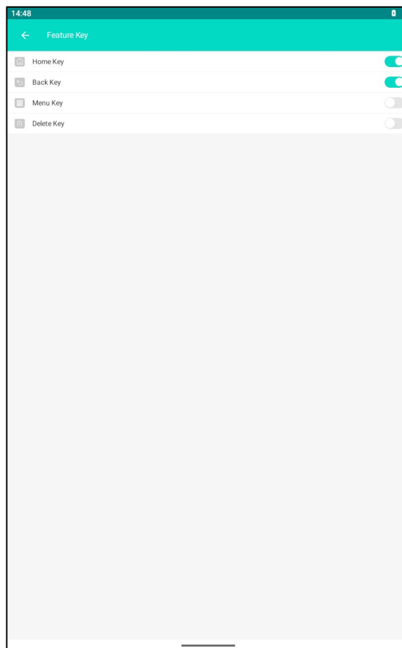
Рисунок 96. Key mask
