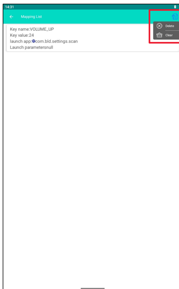
Рисунок 85. Query mapping
