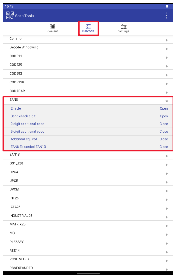
Рисунок 148. EAN8
