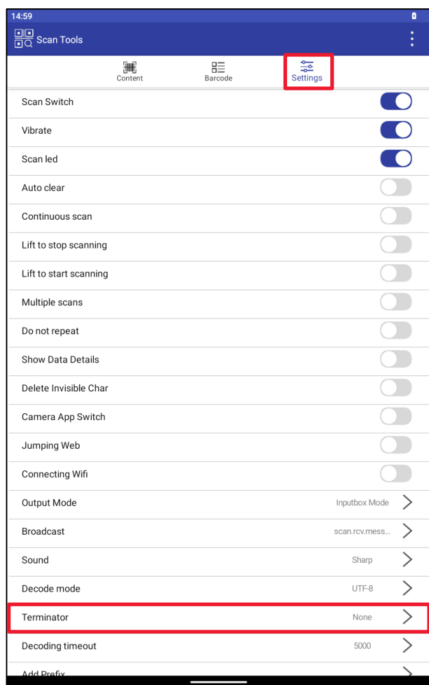
Рисунок 122. Settings. Terminator
