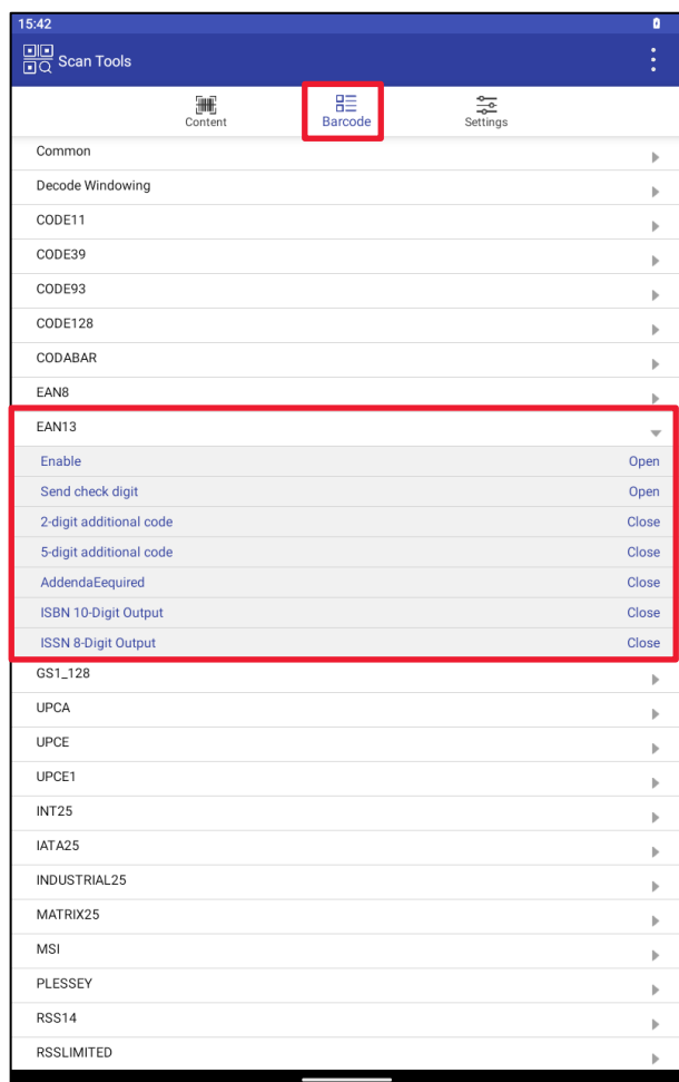
Рисунок 149. EAN13
