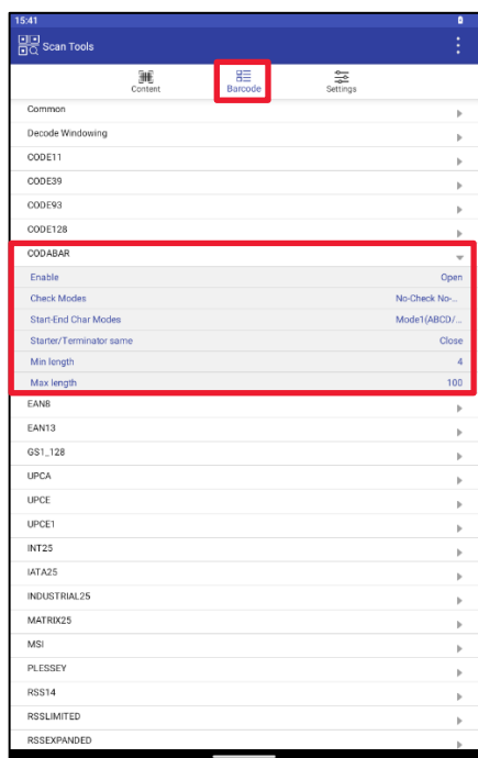
Рисунок 147. CODABAR
