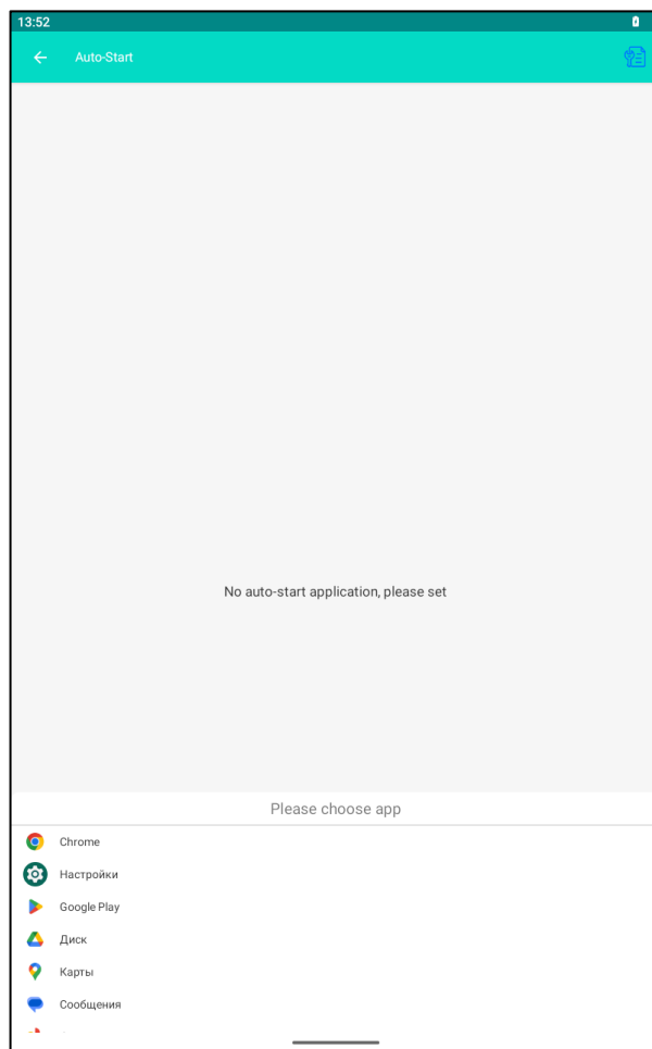
Рисунок 66. Auto-Start
