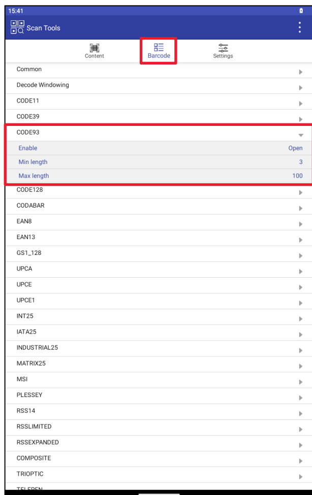
Рисунок 145. CODE93
