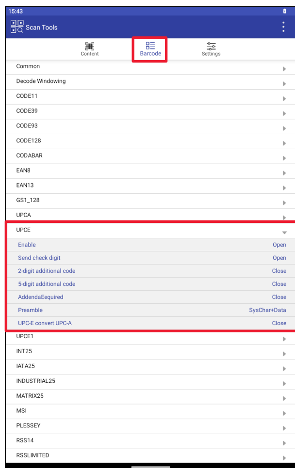
Рисунок 152. UPCE
