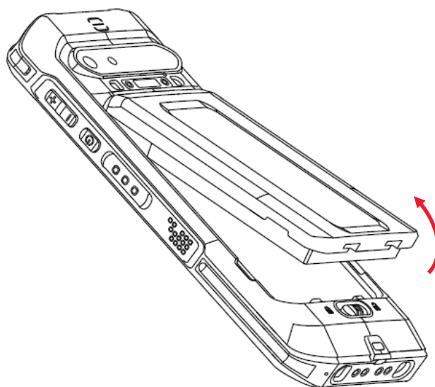
Рисунок 4. Открытие крышки отсека АКБ
