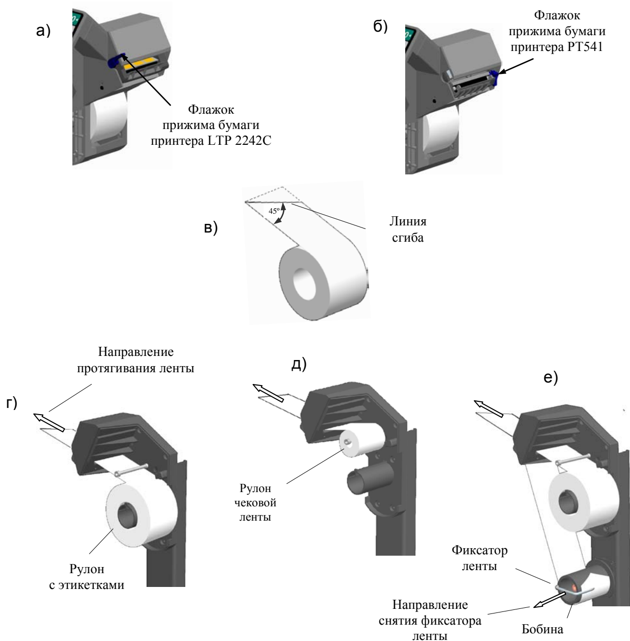
Рис. 6. Установка рулонов
