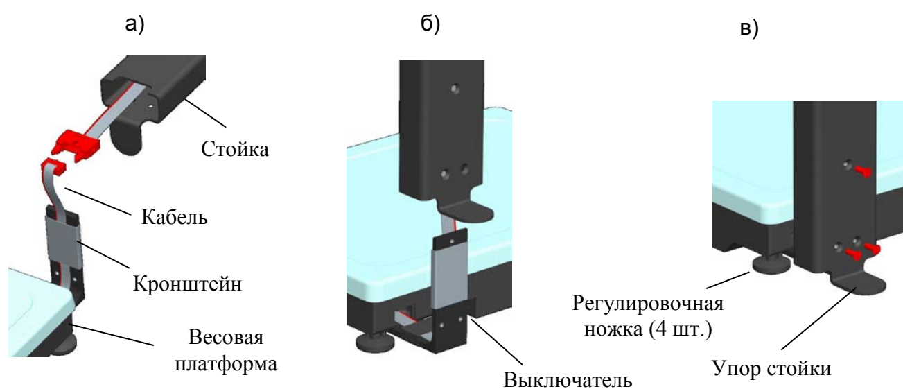
Рис. 4. Сборка
